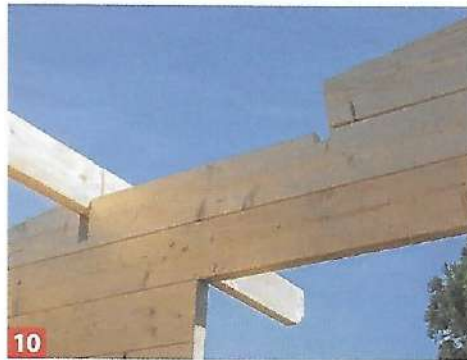
10 Die obersten Bohlen bilden die Schwelle des Dachstuhls und weisen Einkerbungen für die weiteren Dachsparren auf.
